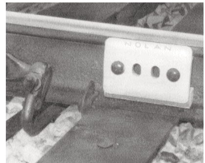
Protectores de agujas de cambio
